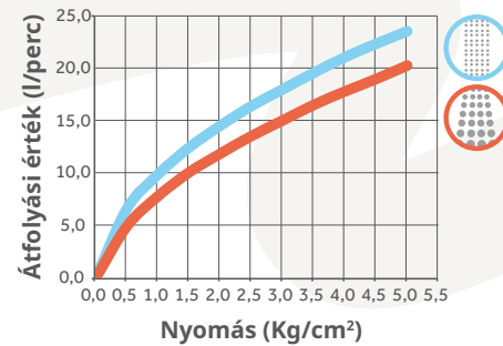
Átfolyási érték és nyomás grafikon
