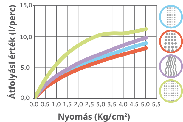
Átfolyási érték és nyomás grafikon
