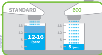
Vízkörmes, víztakarékos perlátör
