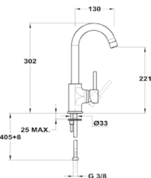
Evo X mosdó csaptelep
