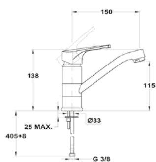
Magasított mosdó csaptelep
