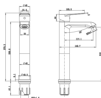
Mosdó csaptelep XL
