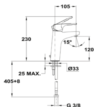
Magasított mosdó csaptelep
