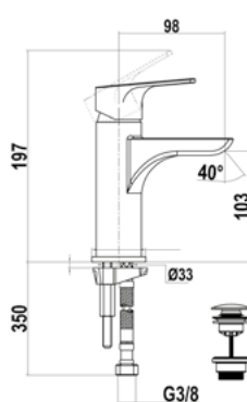
Cascade mosdó csaptelep
