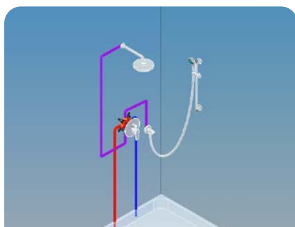
Süllyesztett kétutas csaptelep, zuhanyezett zuhanyrúddal, fali csatlakozós kézzizuhany tartó, zuhanykar, Evo zuhanyfej
