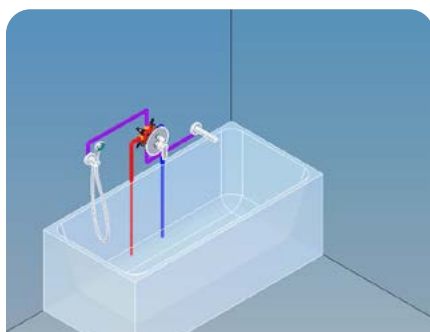
Süllyesztett kétutas csaptelep, fali csatlakozós kézzizuhany tartó, kád kifolyócső
