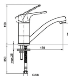
Bojler mosdó csaptelep
