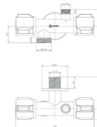
Kerámias sarokszelep 1/2" - 3/8" 163-0040-00
